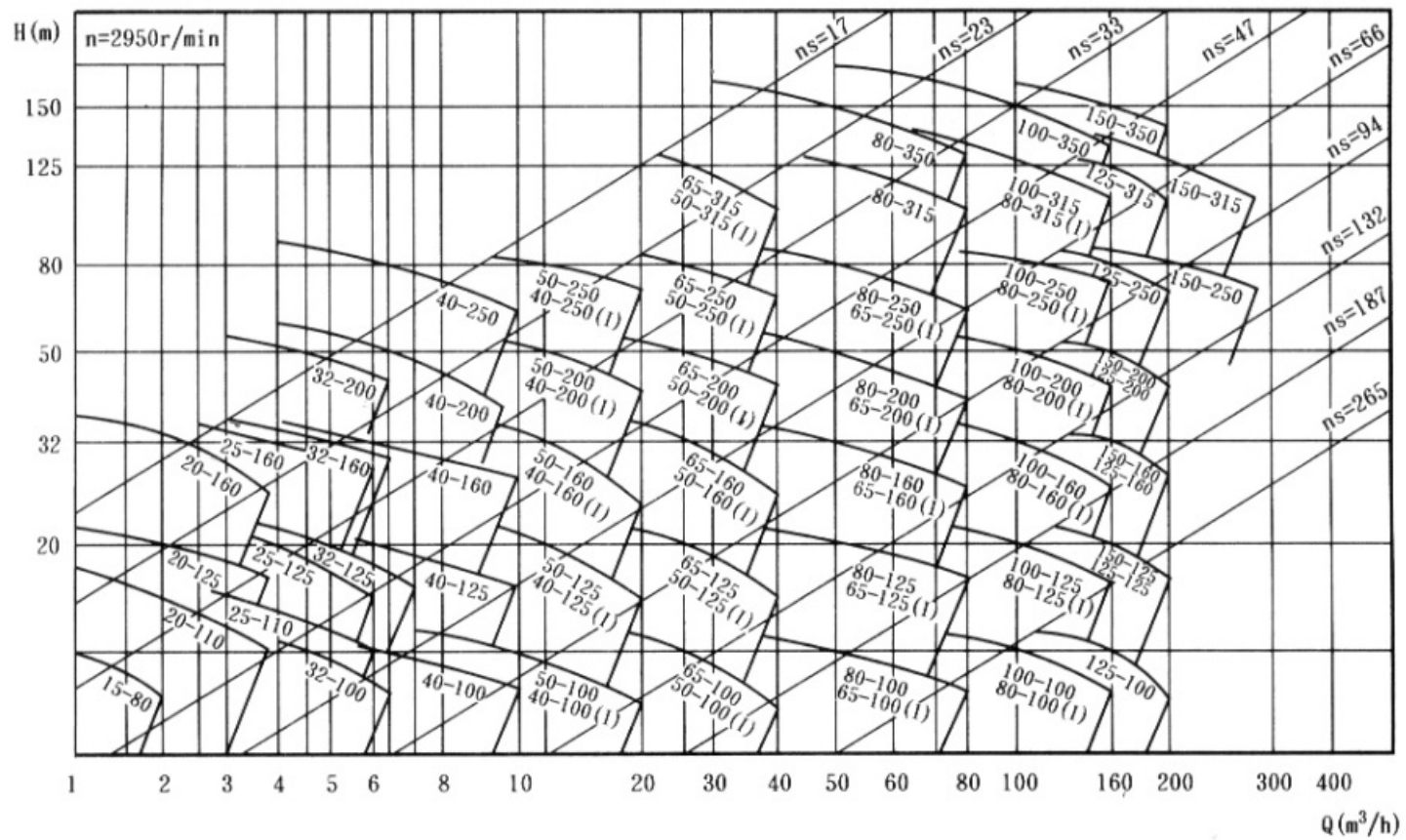
■ TQW、TQWR、TQWH、TQWY、TQWHY型谱图
