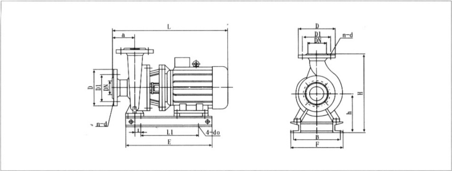
■ TQW、TQWR、TQWH、TQWY、TQWHY型系列泵安装尺寸图表
