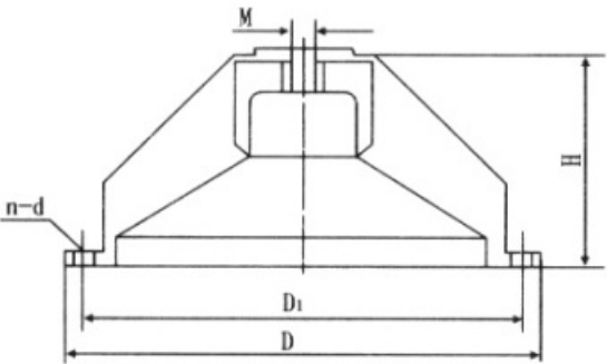
JG型隔振器安装尺寸
