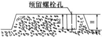
(二)、硬性联接基础图
