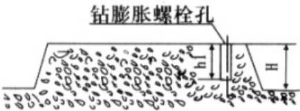
(一)、柔性联接基础图
